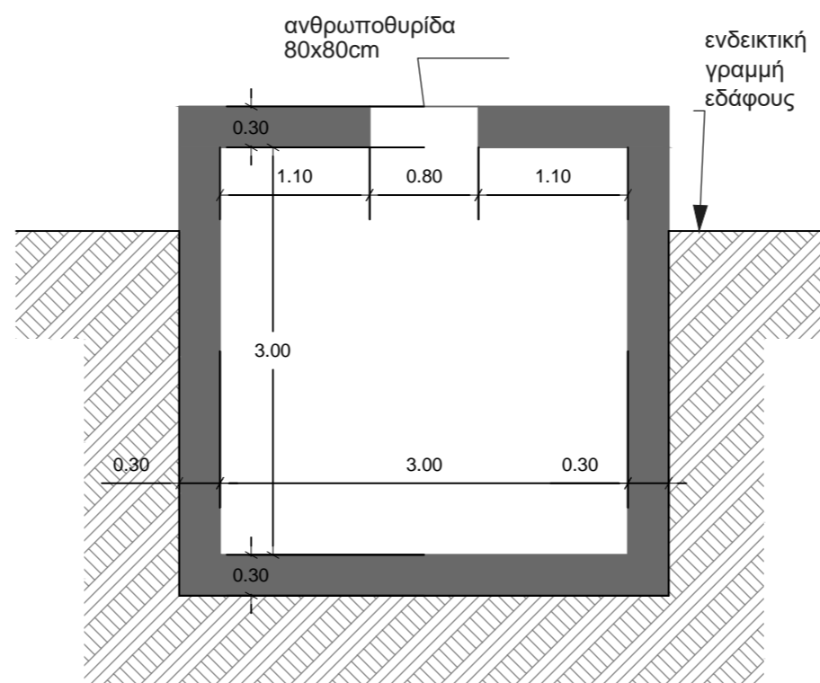
ΤΟΜΗ Β-Β'
