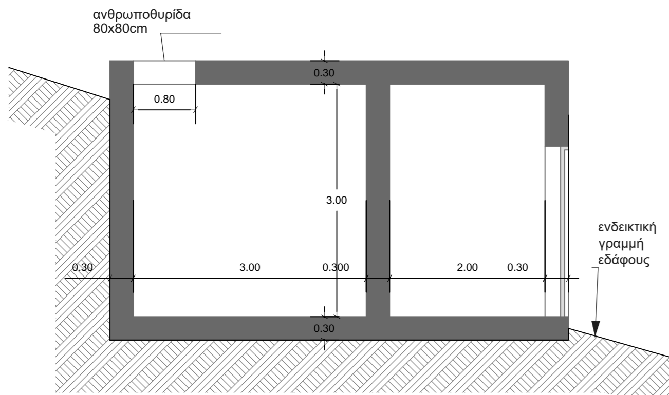
ΤΟΜΗ Α-Α'
