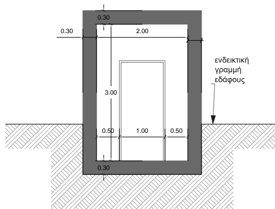
ΤΟΜΗ Γ-Γ'
