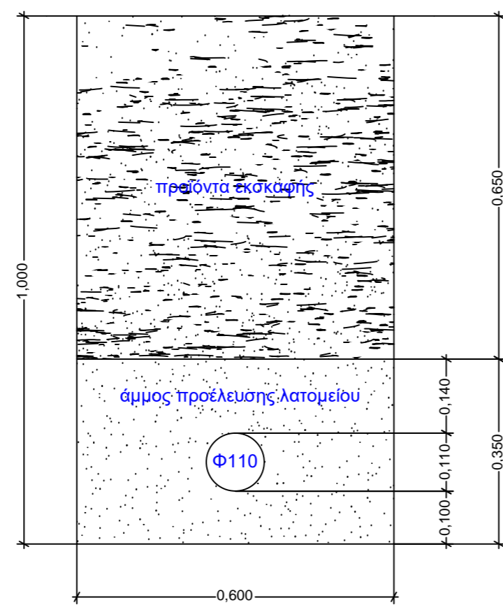
B. Τυπική διατομή σκάμματος στο έρεισμα
