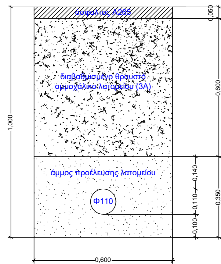
A. Τυπική διατομή σκάμματος στην ασφάλτο
