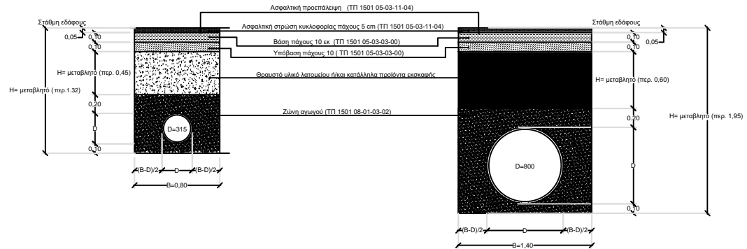
ΣΚΑΜΜΑ ΚΑΤΑΘΛΙΠΤΙΚΟΥ ΑΓΩΓΟΥ Φ315 ΣΕ ΑΣΦΑΛΤΟΣΤΡΩΜΕΝΗ ΟΔΟ ΜΕ ΜΙΑ ΑΣΦΑΛΤΙΚΗ ΣΤΡΩΣΗ
